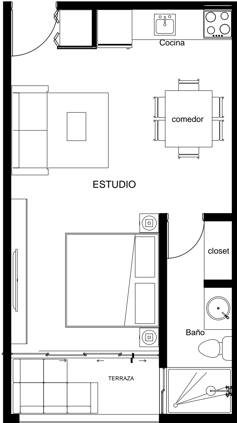
Planta Arquitectónica
